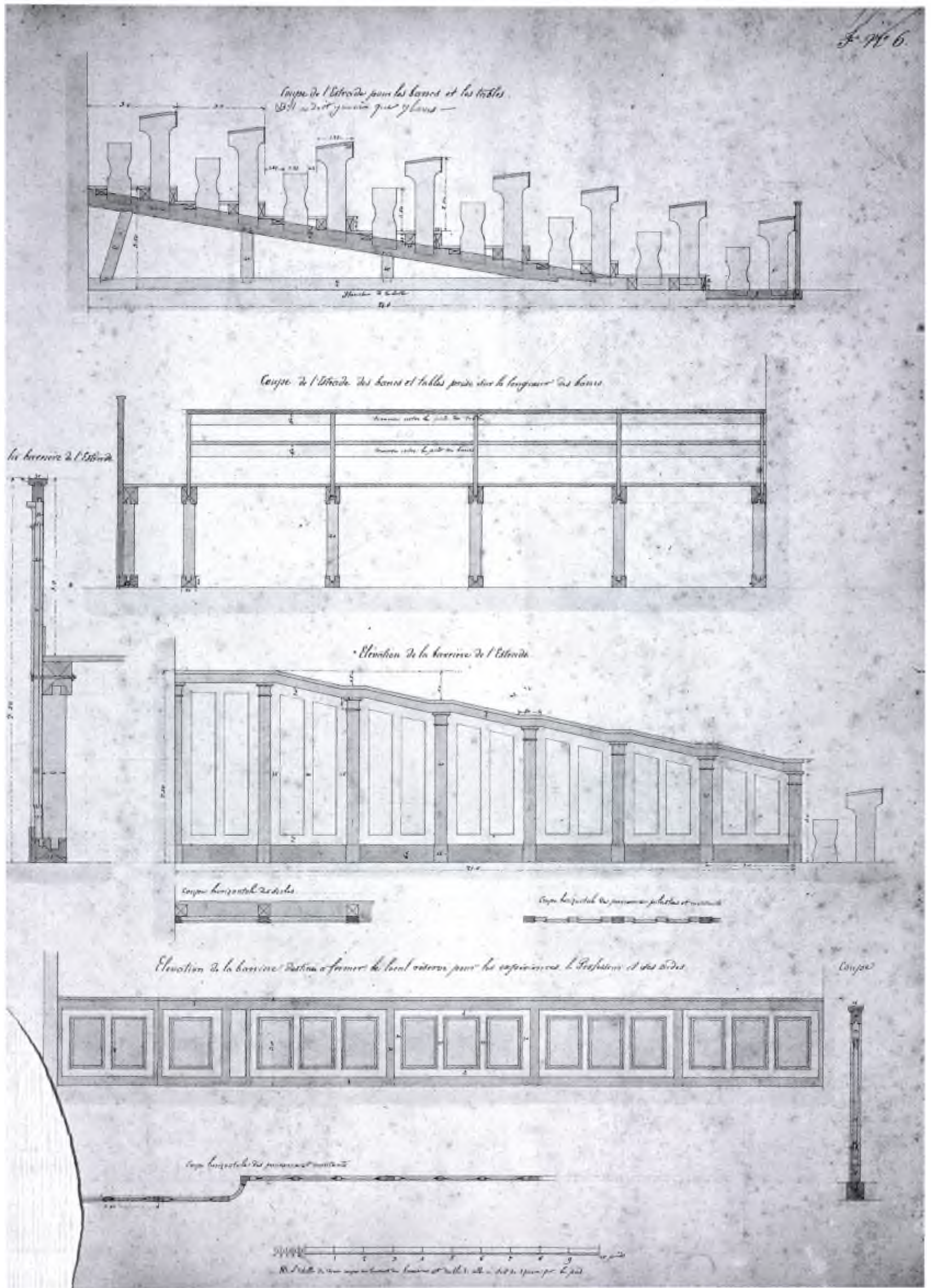
Coupe de l'estrade pour les bancs et les tables, plans pour le Collège académique. (ACV, Bm 9).
